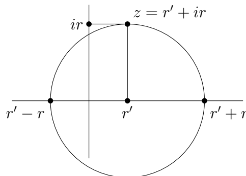
Figura 1.10: Obtención de r' + r y r' - r a partir de r y r' .
