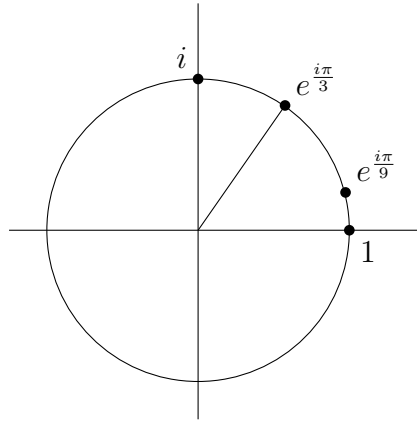
Figura 1.15: Trisección del ángulo de 60^\circ .
